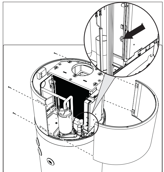
fig. 74- Rimozione del pannello anteriore
