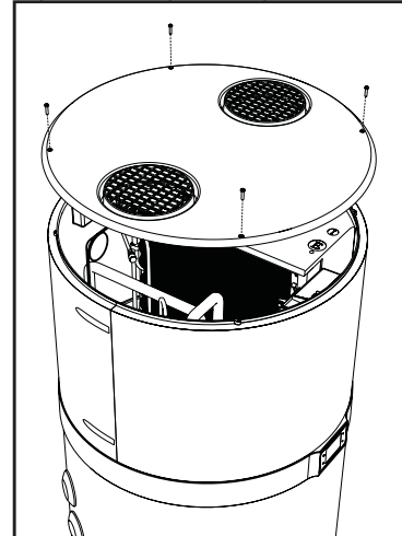
fig. 73- Rimozione del coperchio superiore
