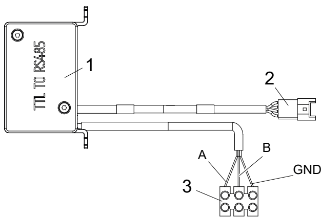
fig. 70 - Kit interfaccia seriale TTL-RS485
