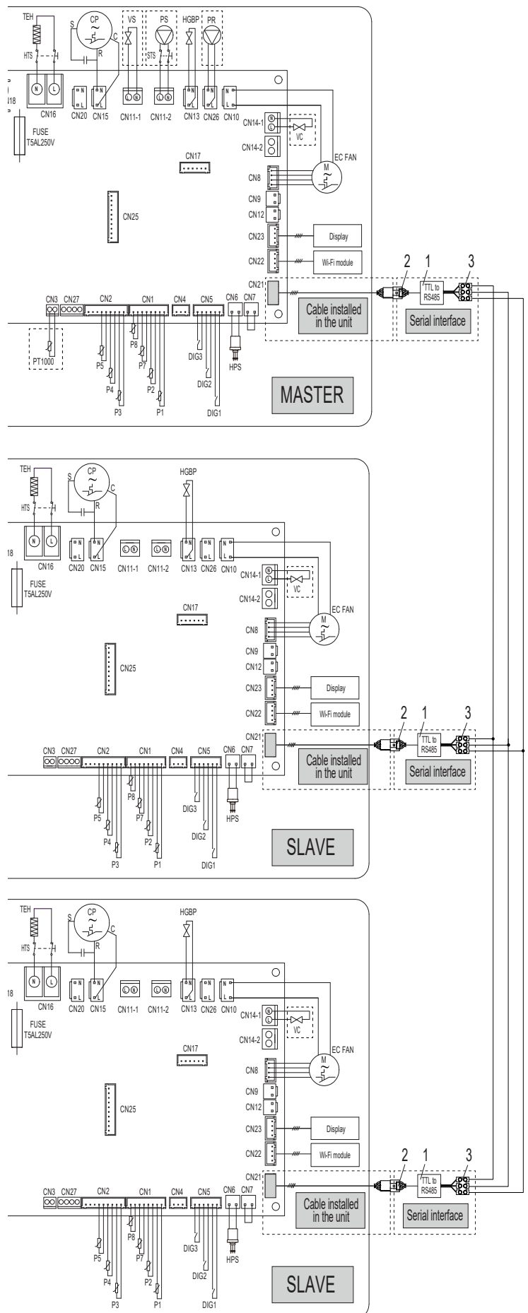
fig. 71 - Schema elettrico cascata
